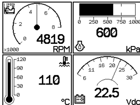
第1頁 常用圖形化錶頭畫面
