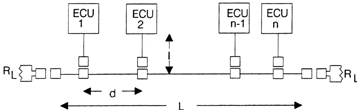
J1939網路拓樸圖
