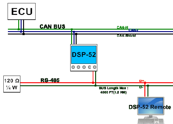
DSP-52 網路連結架構簡圖
