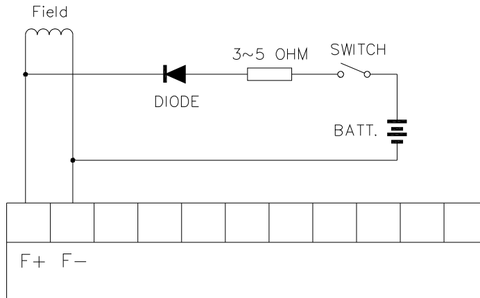
圖五 激磁
