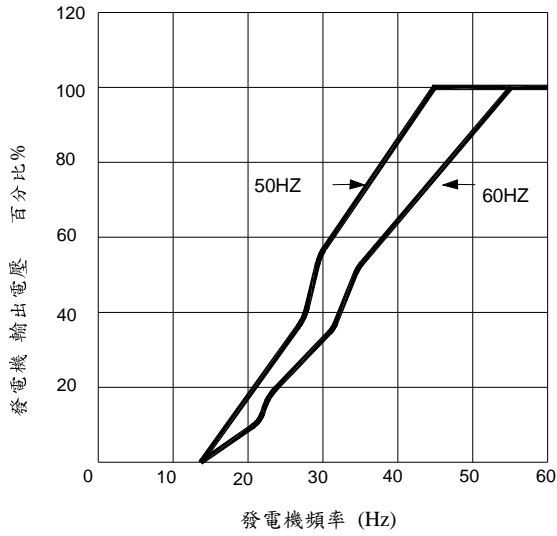
低頻動作曲線 圖二
