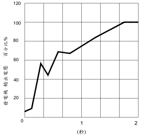
緩慢起動曲線 圖三
