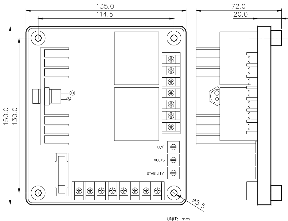
圖一 尺寸與端子、旋鈕
